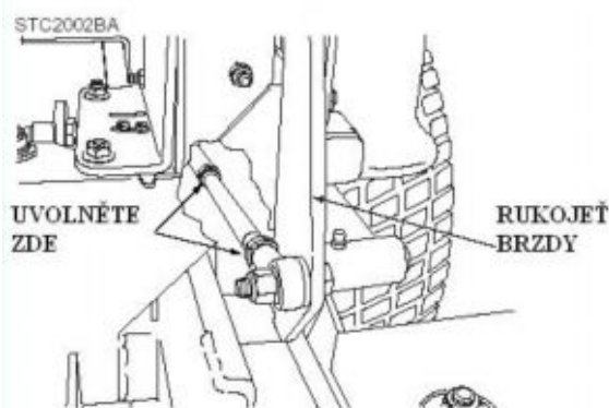
Obr. 6-1 Seřízení brzdy
