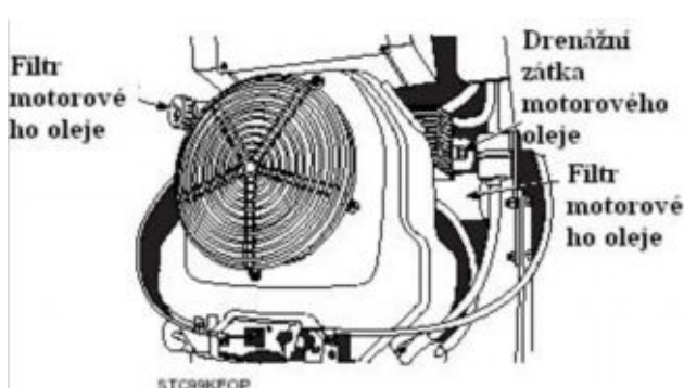
Obr. 7-5 Plnění motorového oleje, měrka, filtr a drenážní zátka
