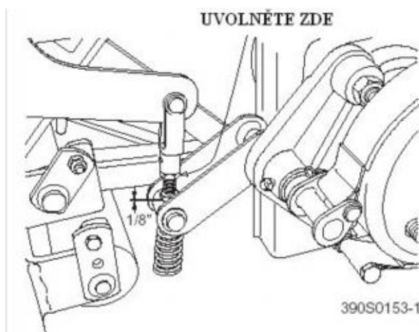
Obr. 6-2 Seřízení táhla brzd
