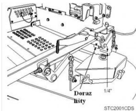
Obr. 6-6 Doraz žacího ústrojí
